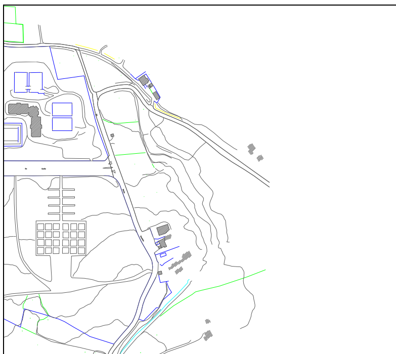
Stralcio aereofotogrammetrico
